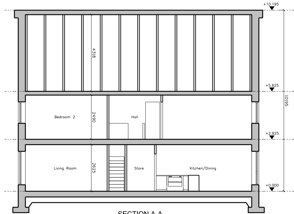
SECTION A-A
